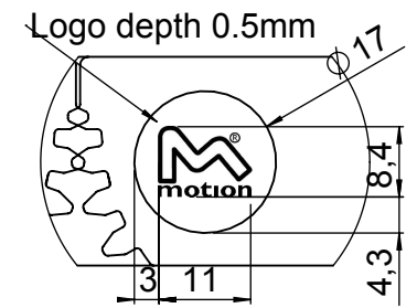
DETTAGLIO A SCALA 1 : 1
