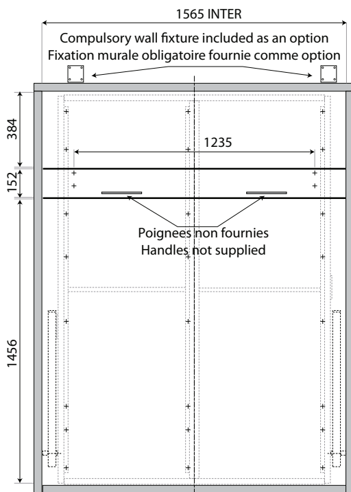
Jeu de plaques métalliques de fixation Set of metal fixtures
